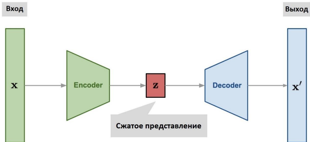
Рисунок 2. Принцип работы архитектур семейства «VAEs».
