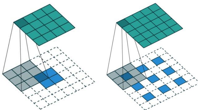
Рисунок 14. Транспонированная свёртка.
