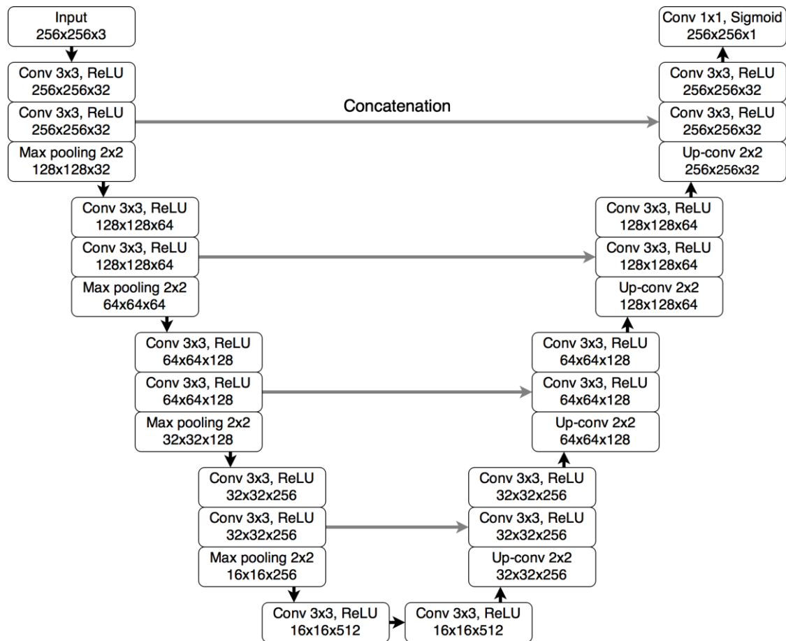
Рисунок 13. Архитектура U-Net.
